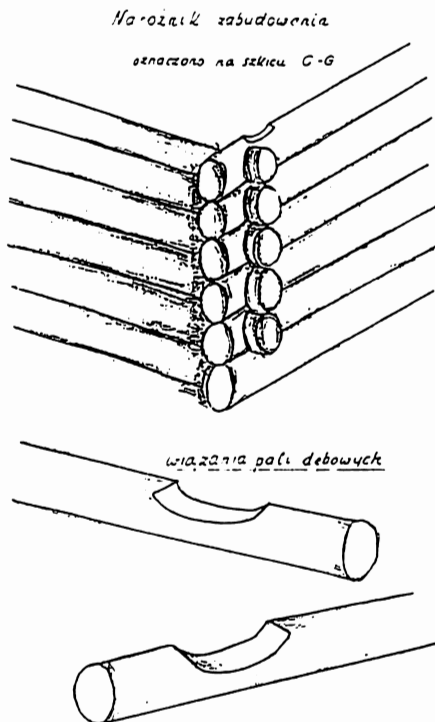
Wiązania odkrytych pali dębowych (rys. Z. Król)
