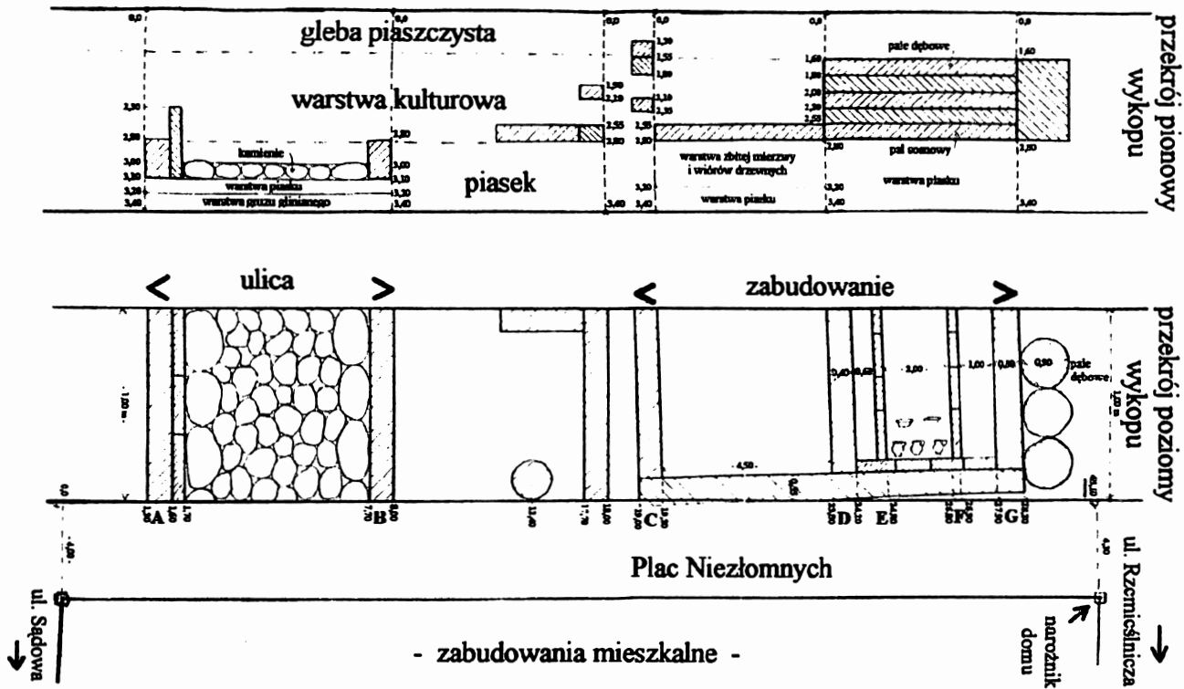
Plan poglądowy znaleziska archeologicznego przy pl. Niezłomnych w Kościanie (rys. Z. Król)
