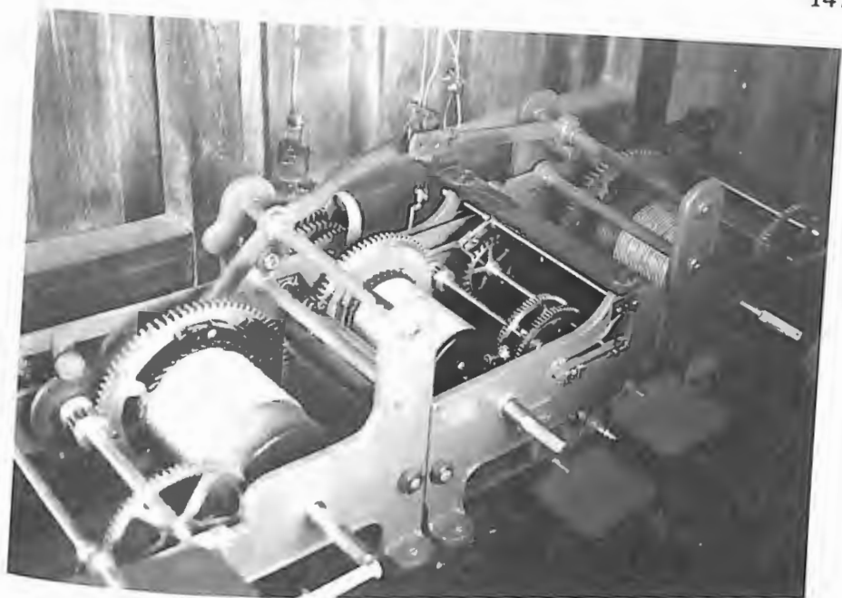
Mechanizm zegara ratuszowego (fot. Z. Garszka)
