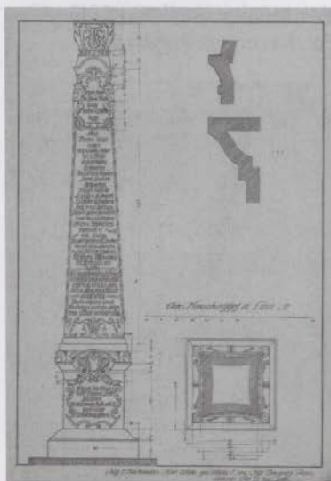
Późnobarokowy nagrobek z cmentarza ewangelickiego w Lesznie. Rysunek E. Barikowiaka i K. Witzke z 1918 r., uczniów Szkoły Budowlanej w Poznaniu. (AWWKZ)
