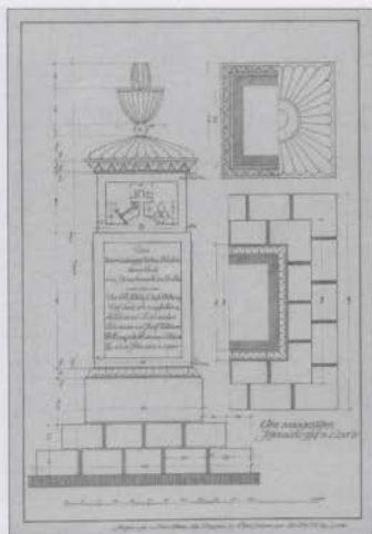
Klasykystyczny nagrobek z dawnego cmentarza ew.-reform. w Lesznie. Rysunek inwentaryzacyjny z 1918 r. (AWWKZ)
