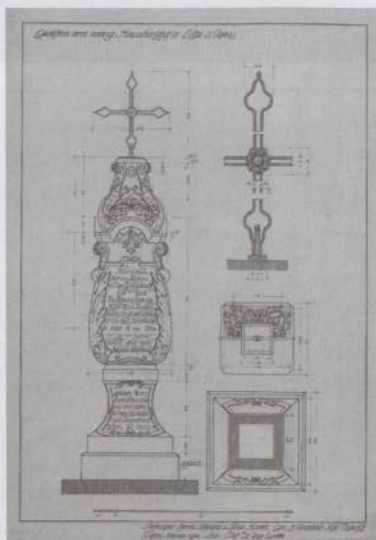
Późnobarokowy nagrobek z cmentarza ewangelickiego w Lesznie. Rysunek inwentaryzacyjny wykonany w 1918 r. (AWWKZ)
