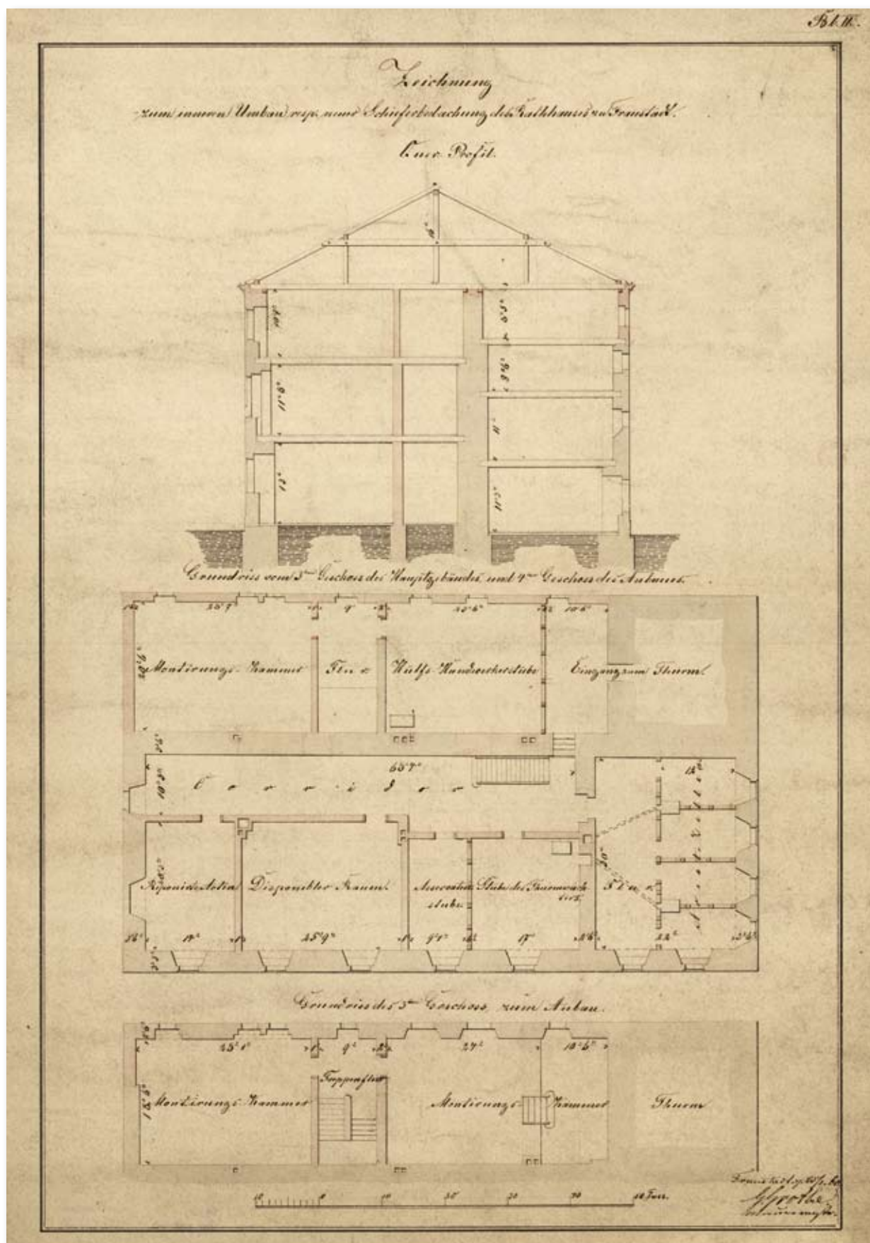
10. Rysunek techniczny układu pomieszczeń wschowskiego ratusza, 1860 r. MZW, nr inw. MZW/K/87. (Reprod. M. Kapała)
