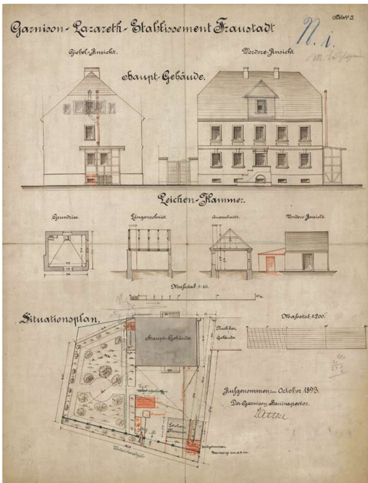
13. Projekt budynku szpitala wojskowego i kostnicy szpitalnej we Wschowie, 1893 r. MZW, nr inw. MZW/K/14. (Reprod. M. Kapala)
